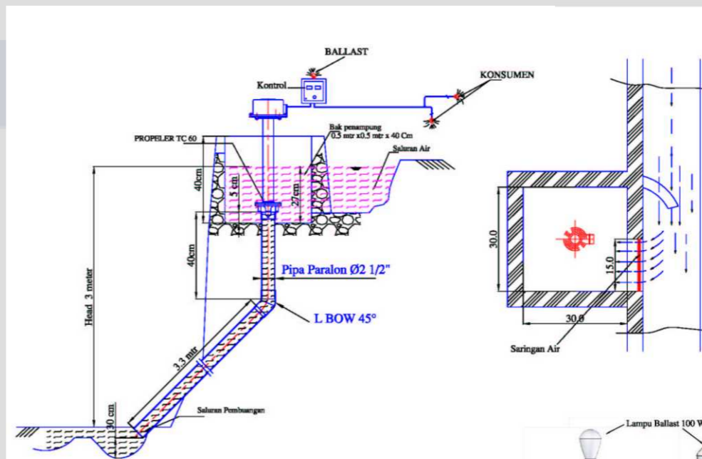
INSTALASI SIPIL
